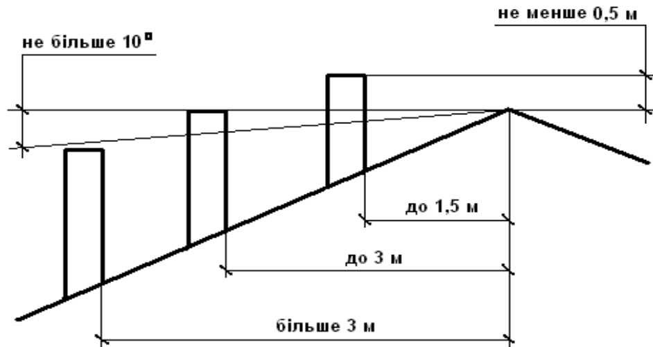
Рисунок 6. Розташування димоходу
