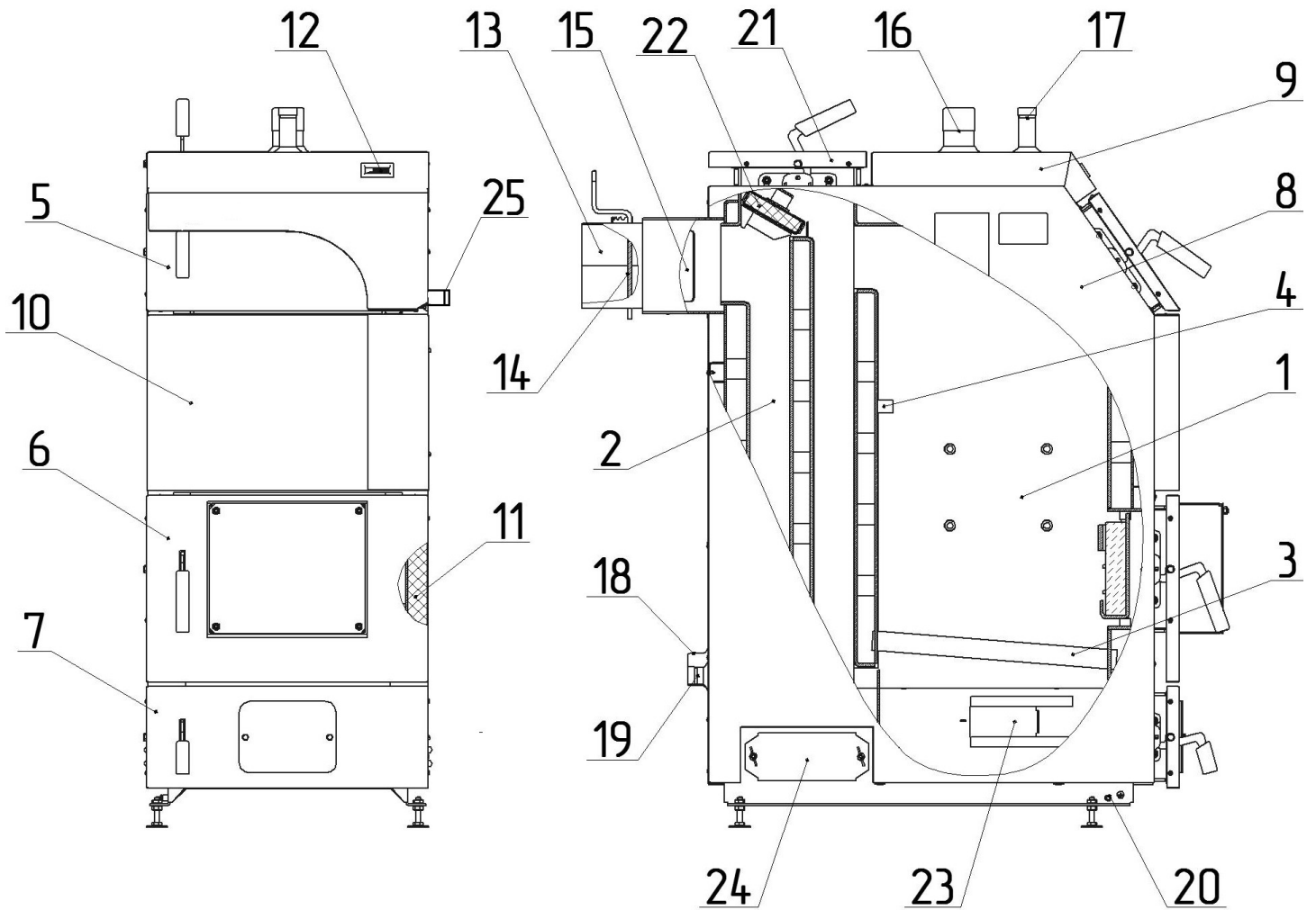
Рисунок 1. Котел опалювальний КТР type V
