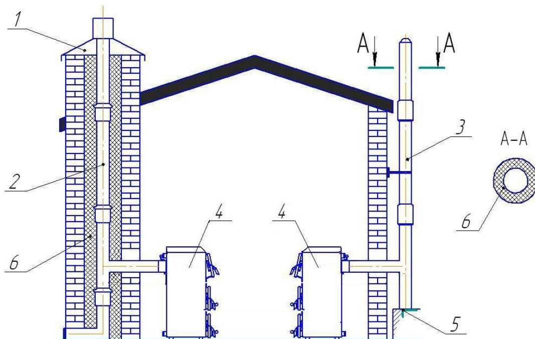
Рисунок 5. Варіанти конструкції димоходу
