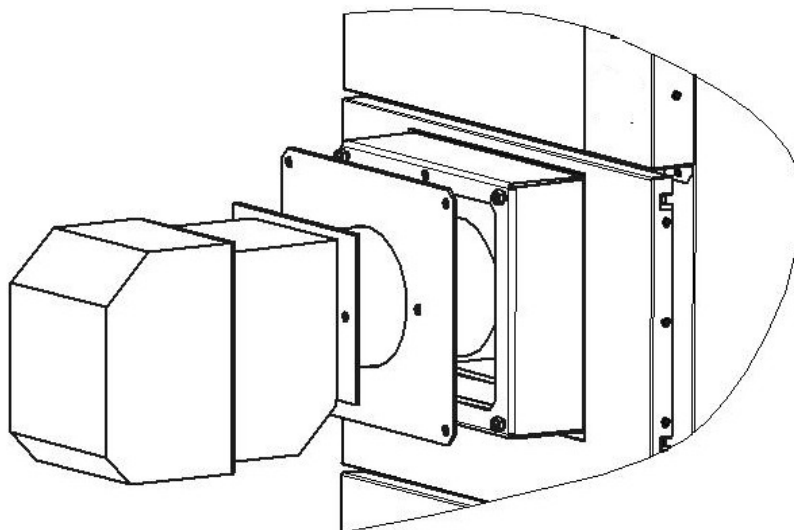
Рисунок 16. Монтаж пальника
