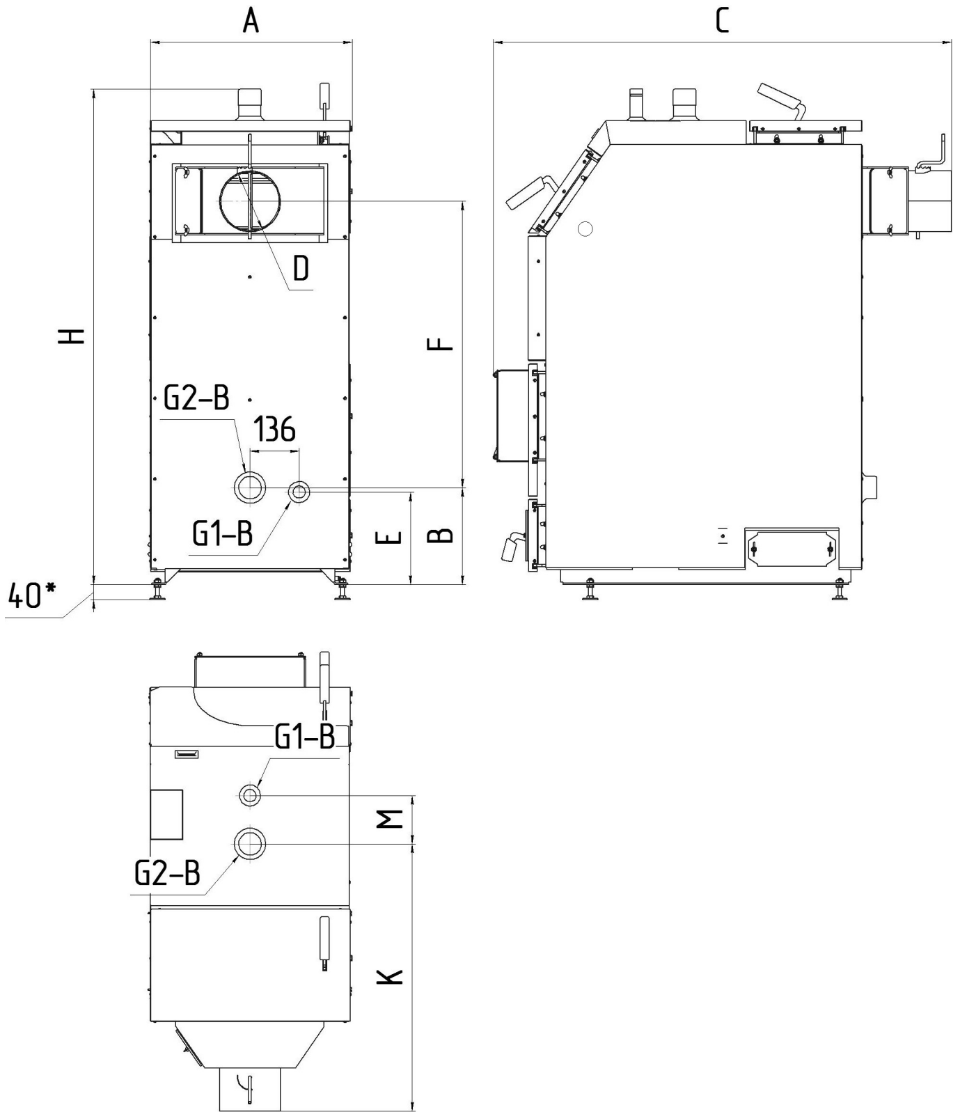
Рисунок 2. Приєднувальні розміри
