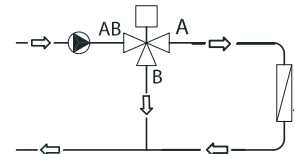
Мал.4. Схема встановлення розділювального клапана на розділення потоку
