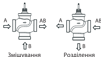
Мал.1. Підключення клапана VRB3 як змішувального, та як розділювального
