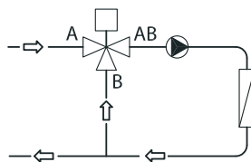
Мал.2. Схема встановлення змішувального клапана на змішування потоків
