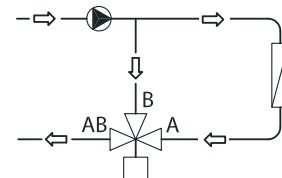
Мал.3. Схема встановлення змішувального клапана на розділення потоків
