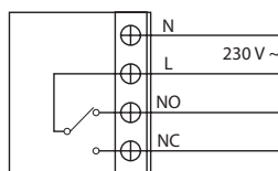
Кімнатний терморегулятор, WT-T
