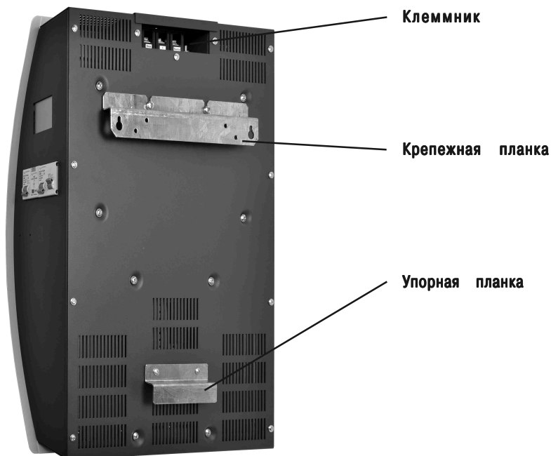
Рис. 2 Стабилизатор вид сзади.
