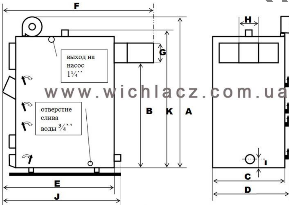
Рисунок 1 – Габаритне креслення котла типу GK-1
