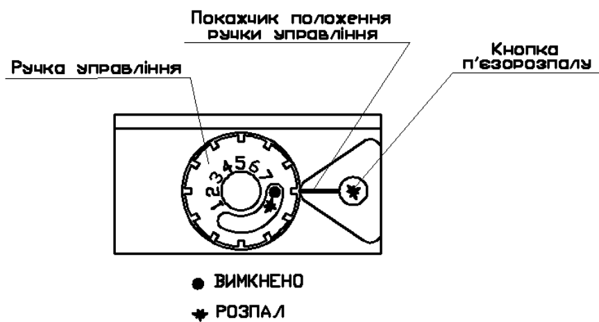
Рисунок 3. Елементи управління газового клапану 630 EUROSIT.
