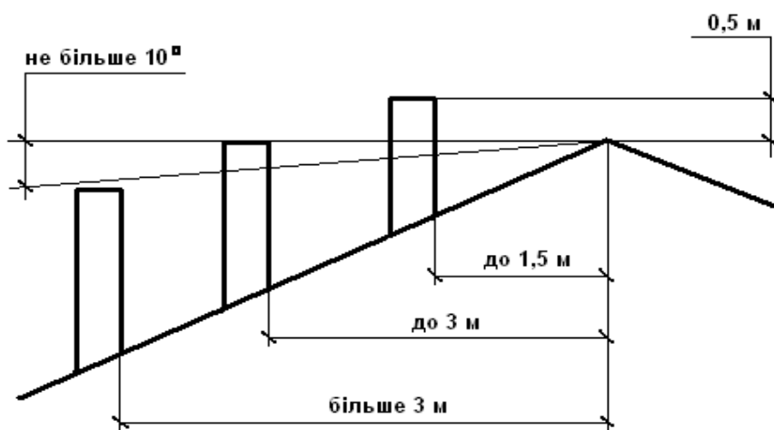
Рисунок 4. Розміщення димоходу
