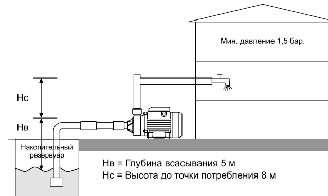
Рис. 1. Типовые схемы водоснабжения с использованием центробежного поверхностного насоса.
