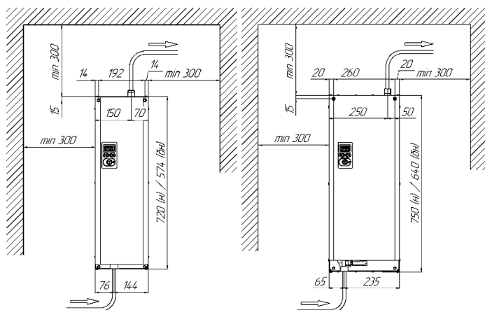
а) Рисунок 2 Розмітка отворів для кріплення а) Котли КОП 4,5 - КОП 15,0; б) Котли КОП 18,0 - КОП 30,0
