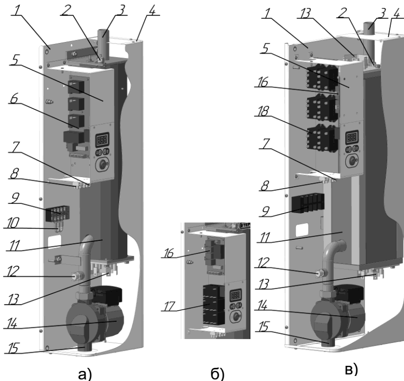
Рисунок 1 Загальний вигляд котла
