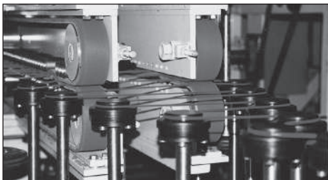
Автоматична лінія виробництва нагрівальних матів
