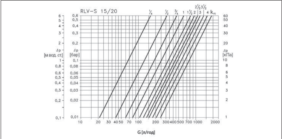
Діаграма пропускної здатності клапанів RLV-S
