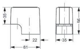
Компактний адаптер для клапанів серії RA (013G5190)
