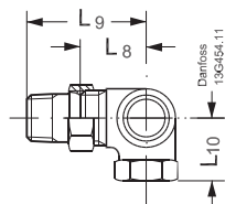
Кутовий клапан для монтажу з правого боку радіатора
