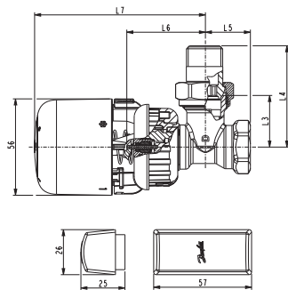
Кутовий клапан з термостатичним елементом Аеро та виносним датчиком
