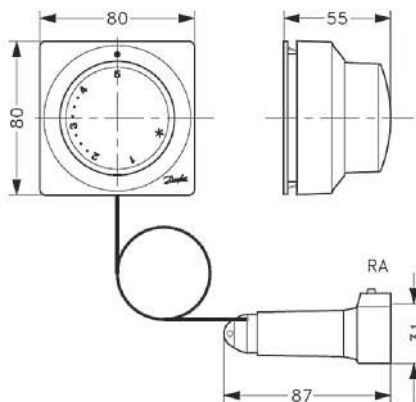
Виносний регулятор температури з адаптером для клапанів серії RA
