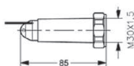
Адаптер для клапанів з різью M30 x 1,5 (013G5194)
