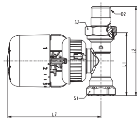
Прямий клапан з термостатичним елементом Aero
