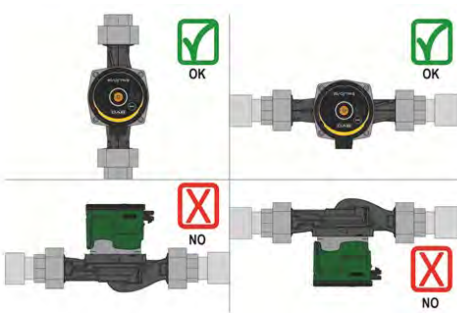
Abb. 3: Montageposition
