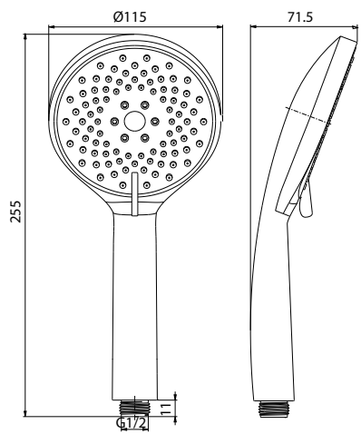
Арт.: 1146460326
