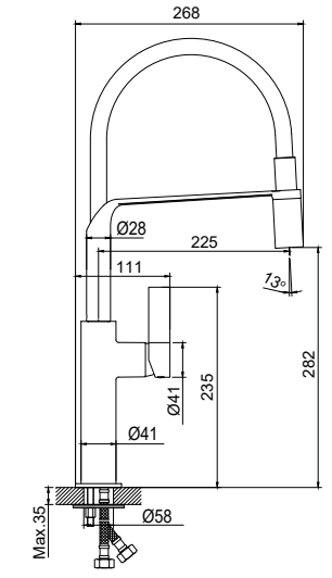
Арт.: 1145441123
