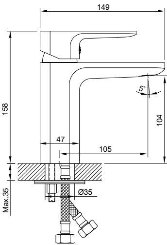
Арт.: 1127330305, 1127330605
