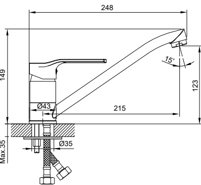
Арт.: 1157310320
