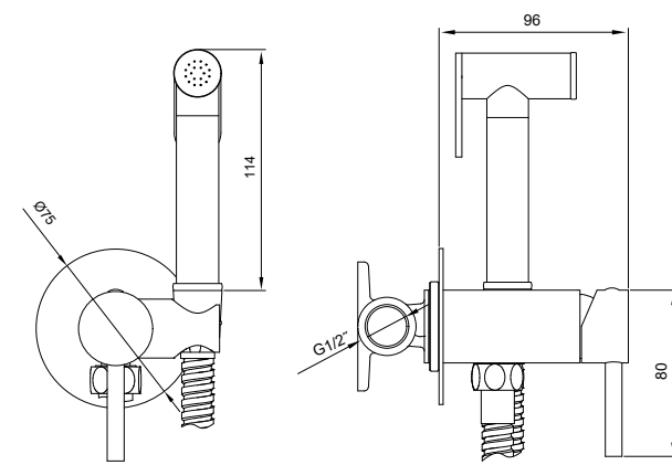
Арт.: 1120400305
