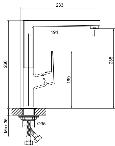
Арт.: 1104310305, 1104310605
