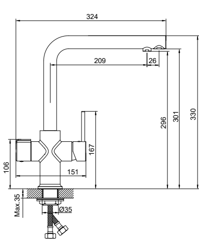
Арт.: 1145420305
