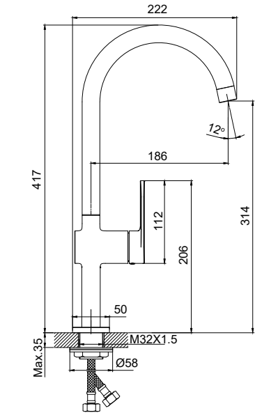
Арт.: 1138310305
