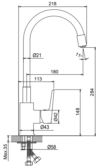
Арт.: 1145441120
