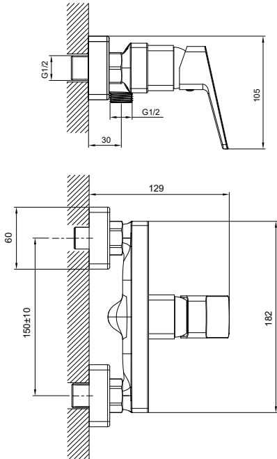
Арт.: 1104320305, 1104320605
