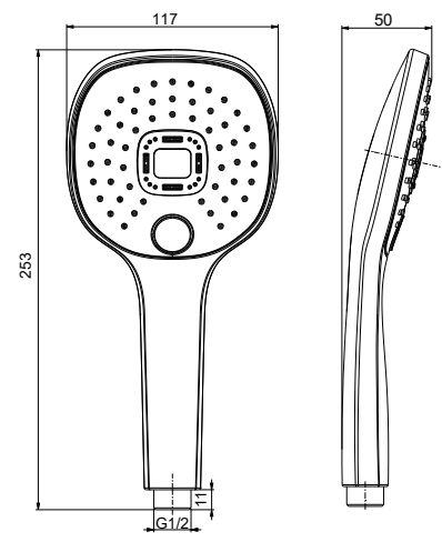
Арт.: 1146461427
