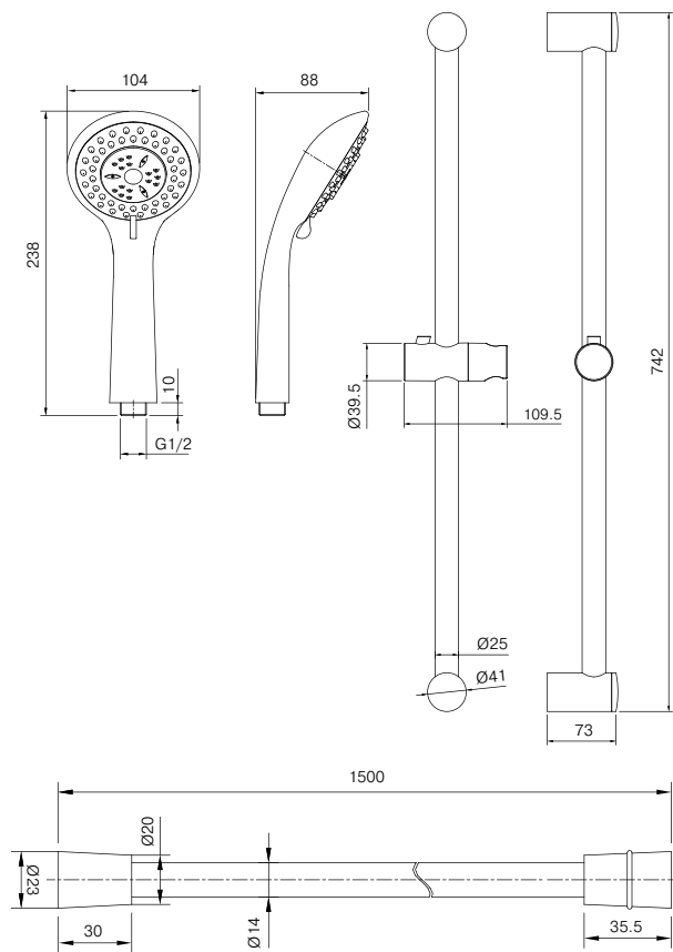
Арт.: 1136360346, 1136360646
