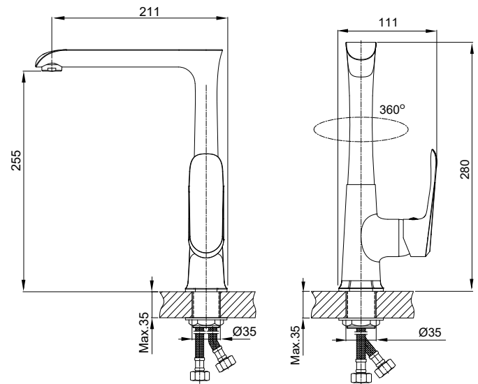
Арт.: 1101310305
