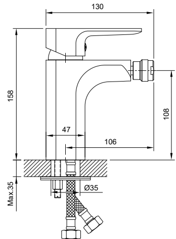
Арт.: 1127350305, 1127350605
