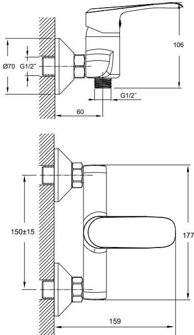
Арт.: 1101320305
