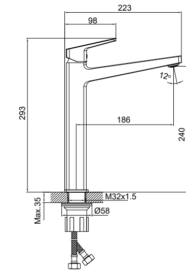
Арт.: 1104350305, 1104350605
