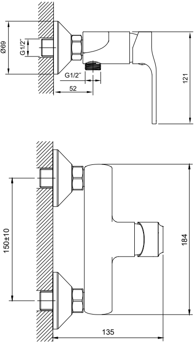
Арт.: 1157320305
