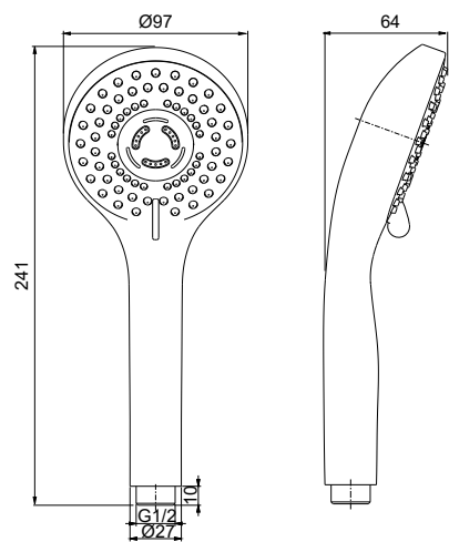
Арт.: 1146461328
