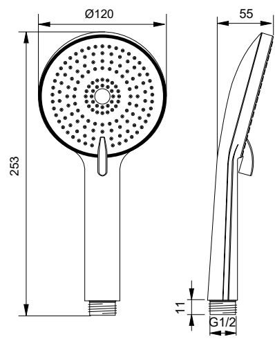
Арт.: 1146460325
