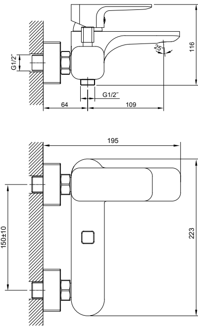
Арт.: 1127300305, 1127300605
