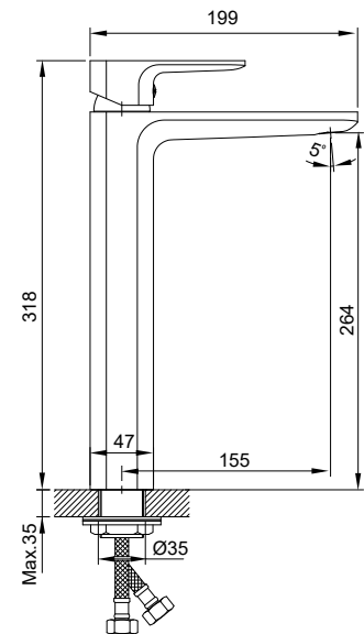
Арт.: 1127340305, 1127340605
