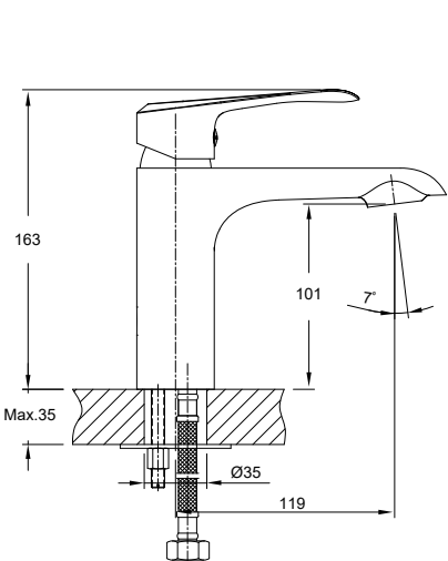
Арт.: 1101330305
