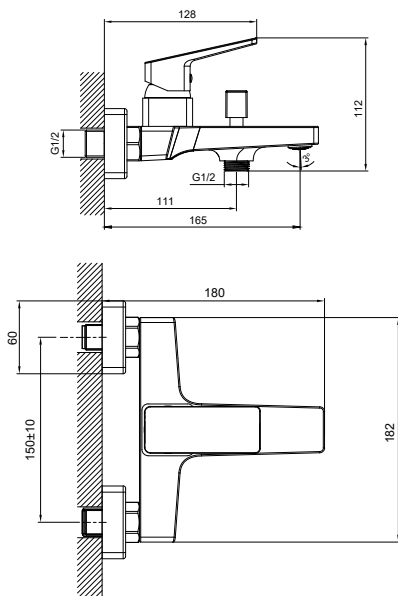
Арт.: 1104300305, 1104300605
