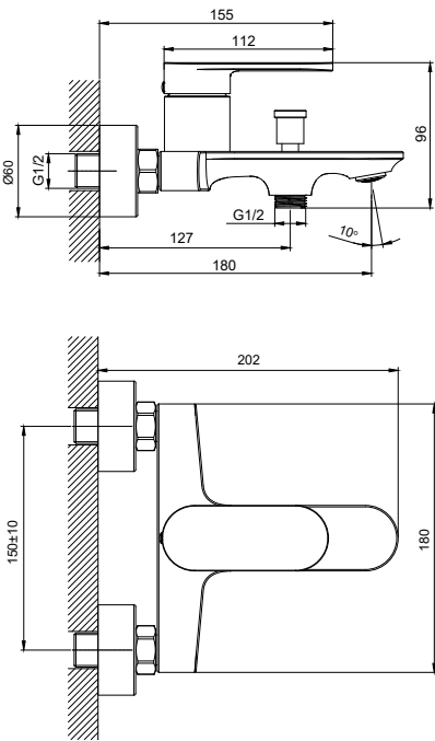
Арт.: 1138300305
