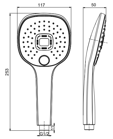
Арт.: 1146460627
