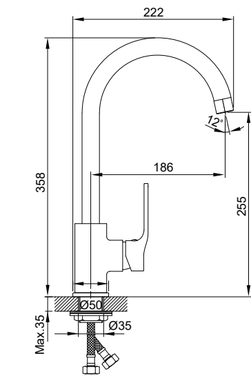
Арт.: 1157310322
