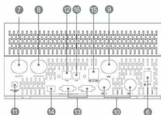
5.2 кВт паралельна модель
