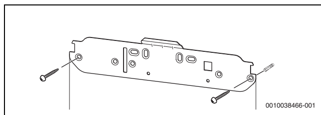
Мал. 28 Монтаж монтажної планки
