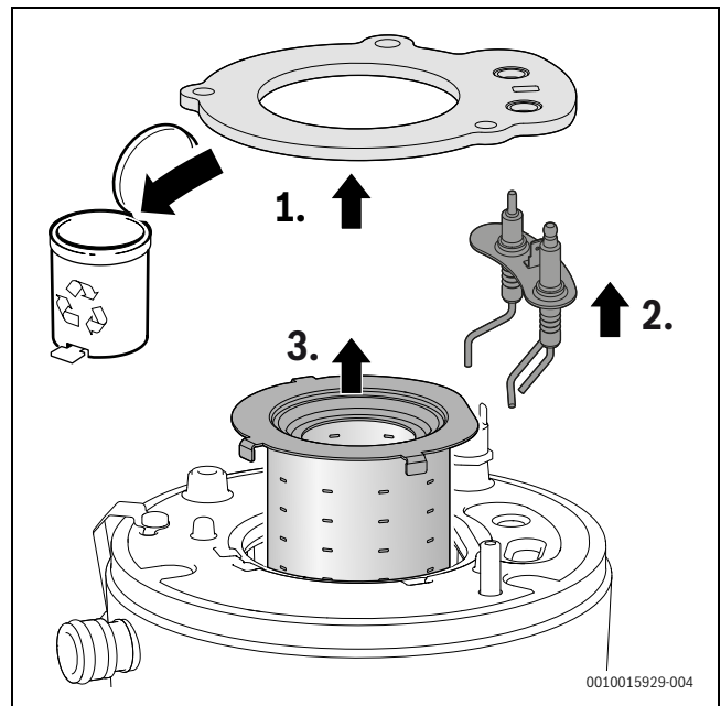
Мал. 54 Виймання пальника
